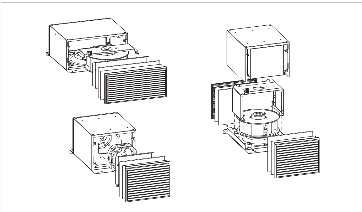
Diferentes modelos de ventilador de techo
